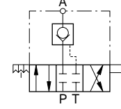
Centro Cerrado
