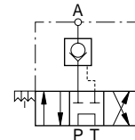
Tandem-Mittelstellung
