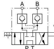
Tandem-Mittelstellung
