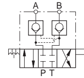
Centro Cerrado
