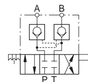
Centro tandem
