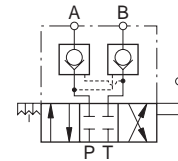
Centro fechado
