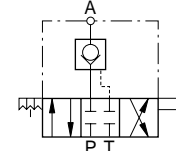
Geschlossene Mittelstellung
