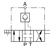
Centro fechado
