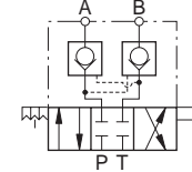
Geschlossene Mittelstellung
