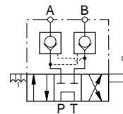
Centro tandem
