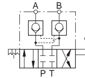
Centre fermé
