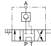
Tandem-Mittelstellung
